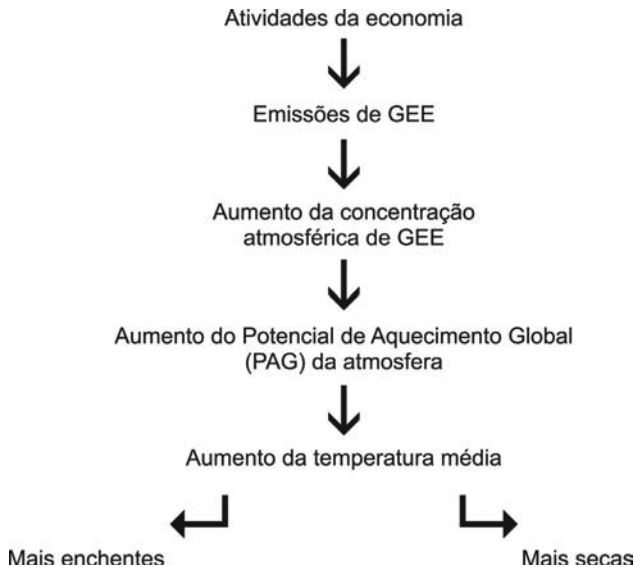
Figura 1 - Cadeia de eventos relacionados às mudanças climáticas. Fonte: AMBRIZZI, 2007.
