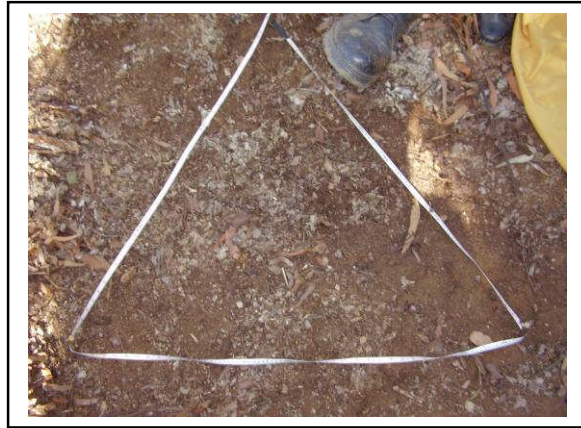
Figura 5 - Forma de triângulo para os testes com infiltrômetro, na Bacia Hidrográfica do Córrego Zerrede, Timóteo-MG, 2008.
