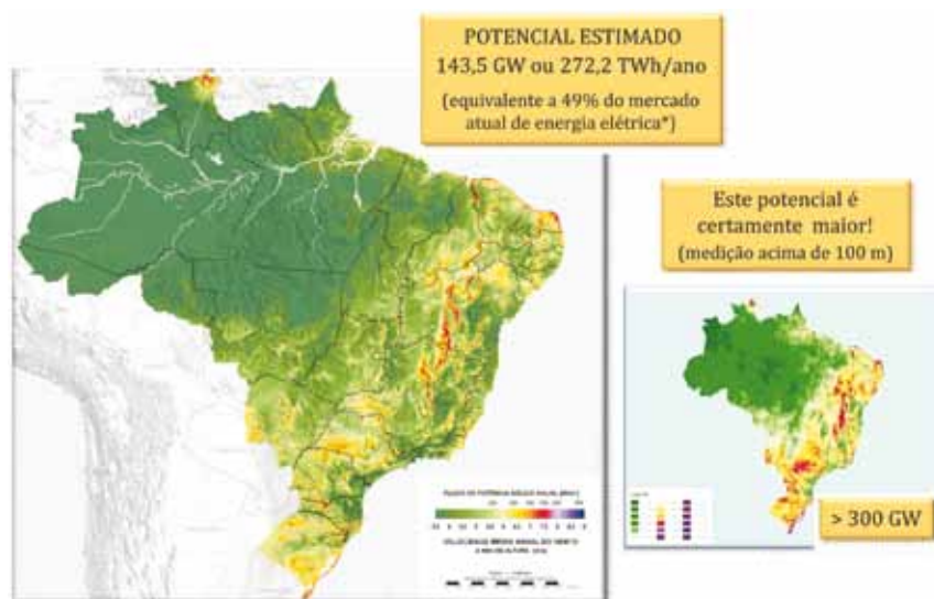
Figura 8. Distribuição Geográfica do Potencial Eólico Brasileiro
