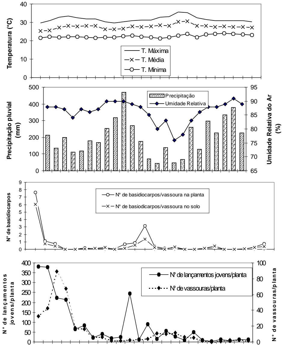
FIG. 1. Número de lançamentos jovens e de vassouras verdes/planta (A), produção de basidiocarpos/vassoura na planta e no solo (A), precipitação pluvial (mm) e umidade relativa do ar (%) e (C) e temperatura (°C) máxima, média e mínima (D), no período de junho de 1996 e maio de 1998, em Manaus-AM.
