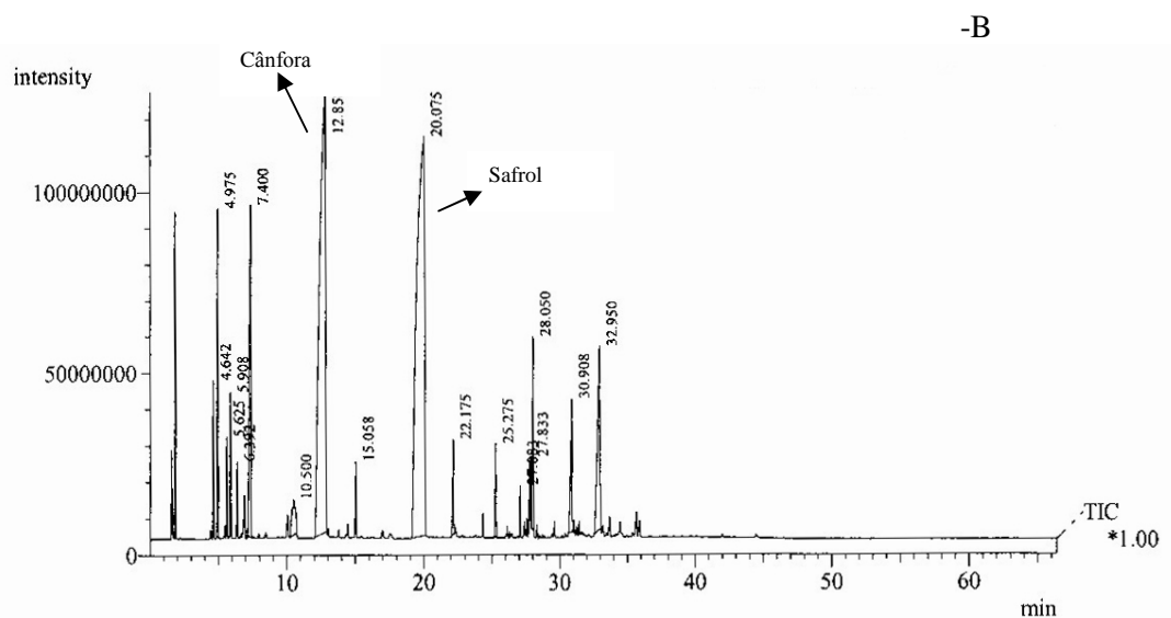
Figura 3.9 - Cromatogramas das amostras da primavera: Omissão de Mg; Omissão de S e Omissão de B da Ocotea odorifera .
