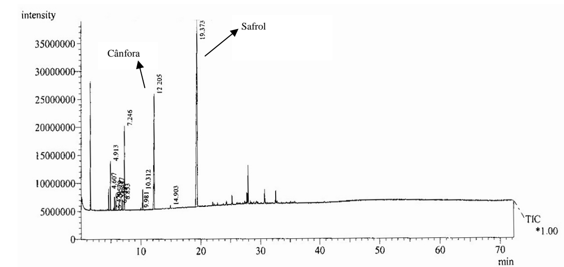
Figura 3.8 - Cromatogramas das amostras da primavera: Omissão de P; Omissão de K e Omissão de Ca da Ocotea odorifera .
