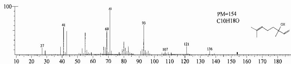
Figura 3.12 - Espectros de massa do p-cimeno (1), o-cimeno (2), limoneno (3), \alpha -terpineol (4) e linalol (5) do óleo das folhas da primavera de Ocotea odorifera .
