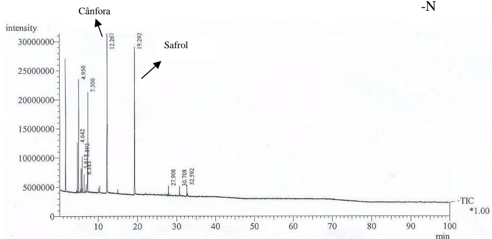
Figura 3.7 - Cromatogramas das amostras da primavera: Controle, Adubação completa e Omissão de N da Ocotea odorifera .
