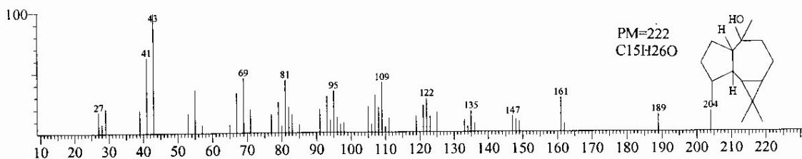
Figura 3.13 - Espectros de massa da cânfora (1), safrol (2), germacreno (3), espatulenol (4) e globulol (5) do óleo das folhas da primavera de Ocotea odorifera .
