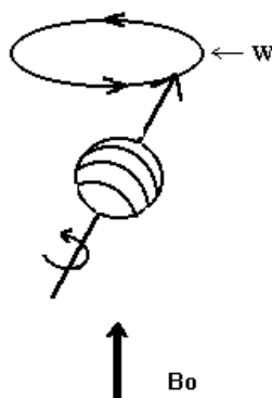
Figura 1. Diagrama do movimento de precessão do spin em torno do campo magnético B_0 .
