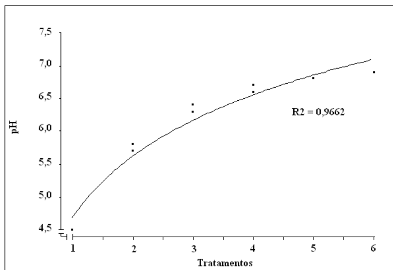
Figura 6. Curva de neutralização do solo com calcário, onde, tratamento 1: 0 Mg de calcário/ha, tratamento 2: 1 Mg de calcário/ha, tratamento 3: 2 Mg de calcário/ha, tratamento 4: 3 Mg de calcário/ha, tratamento 5: 4 Mg de calcário/ha e tratamento 6: 5 Mg de calcário/ha
