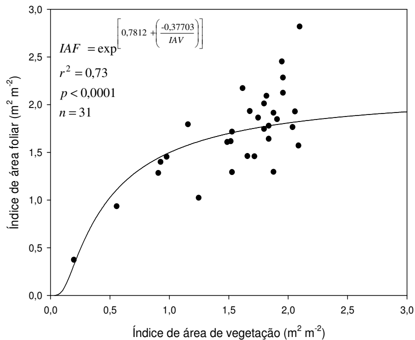
Figura 17 – Equação de calibração para estimativa do índice de área foliar (IAF) em função do índice de área de vegetação (IAV) obtido pelo programa Hemisfer . Os pontos representam as 31 amostras destrutivas para obtenção do IAF real.
