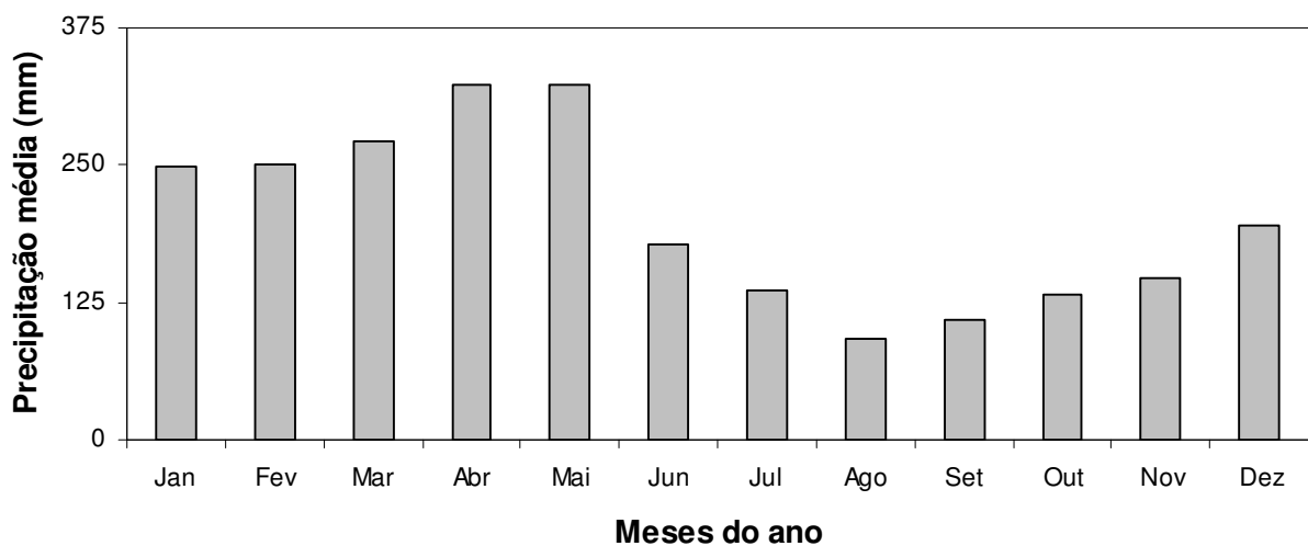
Figura 2 – Pluviometria média mensal (1986 – 2004) da Estação da CEPLAC (Comissão Executiva do Plano da Lavoura Cacaueira), localizada no km 50 da BR 174 (02° 33' S e 60° 01' W), Manaus, Amazonas.
